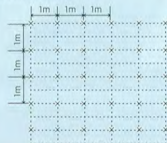
ケモnonネット 止め釘打設図
